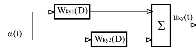
Рисунок 1. Двухзвенная система
