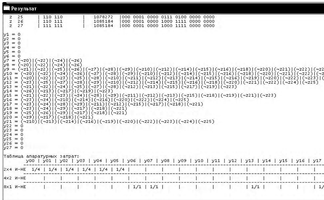
Рис. 4. Выведение результирующей функции и таблицы аппаратных затрат
