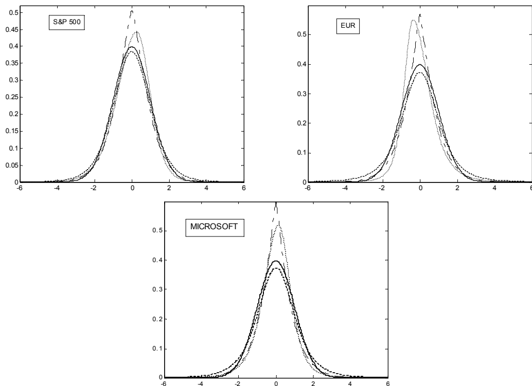
Рис. 4. Графики теоретических функций плотности распределения доходностей S&P 500, EUR, Microsoft ( ——— - плотность нормального распределения, - - - -распределения Стьюдента, - . - . - распределения Хансена , ..... - распределения GED)
