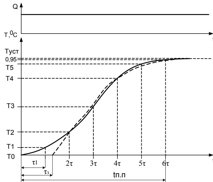
Рис. 1. Переходная функция исследуемого объекта
