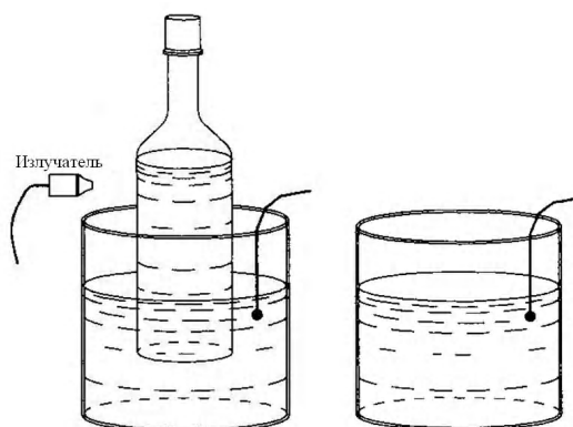
Рис. 1. Схема дистанционного измерения концентрации раствора
