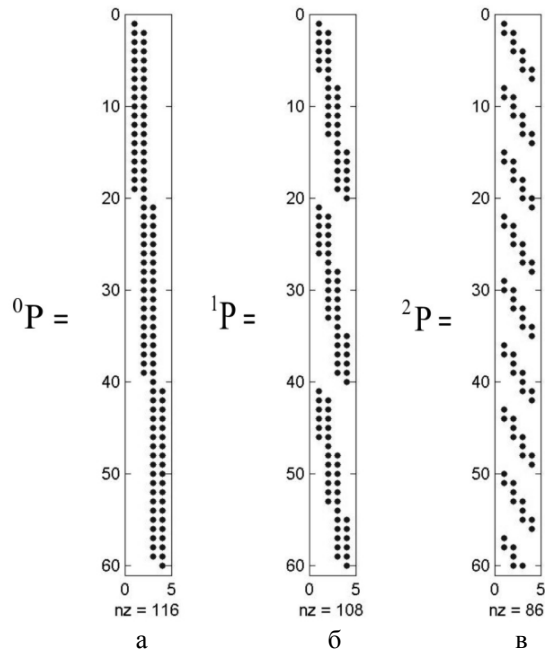
Рис. 1. Внутрішня структура матриць планування: а – нульового масштабу; б – першого масштабу; в – другого масштабу
