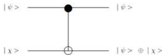
Рис. 2. Контролируемое НЕ
