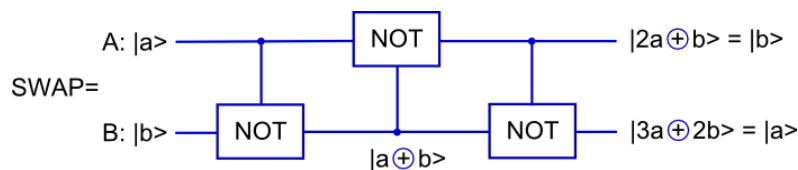
Рис. 3. Оператор SWAP
