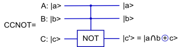
Рис. 4. Вентиль Тоффоли
