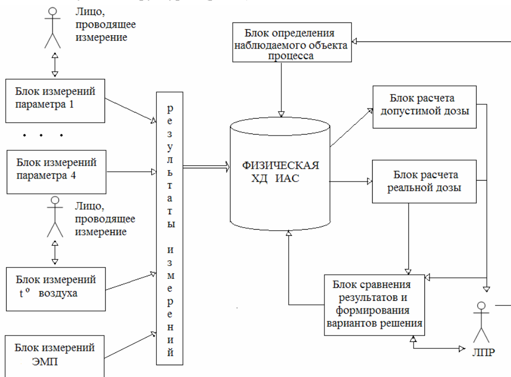
Рис. 3. Схема структуры информационно-аналитической системы управления безопасностью производства
