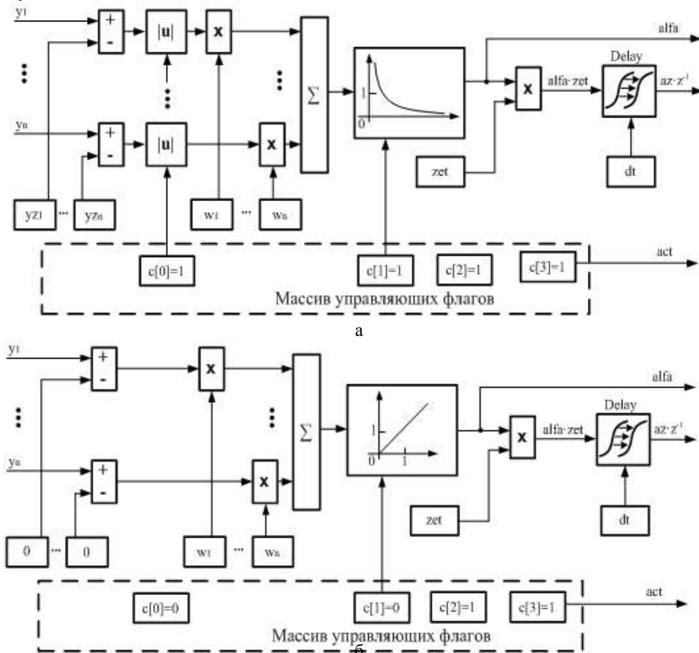
Рис. 1. Структурная схема агента: а – вариант распознавания вектора (флаги c[0]=1 и c[1]=1 ); б – вариант для вычисления функциональной зависимости (флаги c[0]=0 и c[1]=0 )
