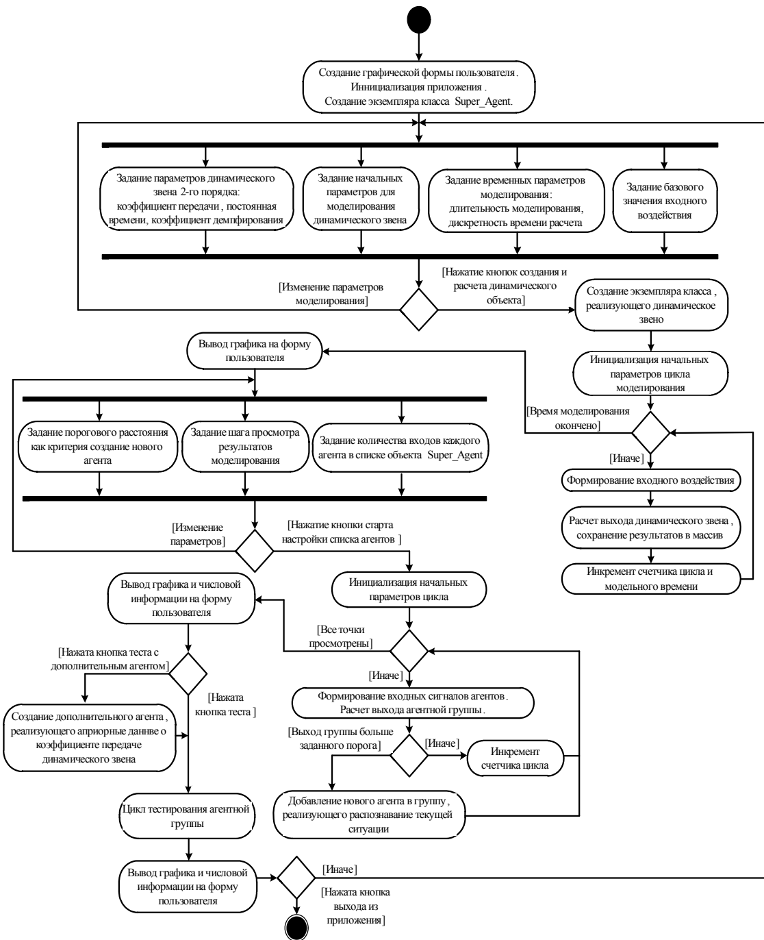
Рис. 5. UML-диаграмма активности работы тестового приложения, использующего агентный супер-визор
