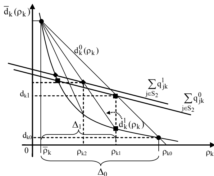
Рис. 2. Иллюстрация процесса приближения к нулю функции условия (16)
