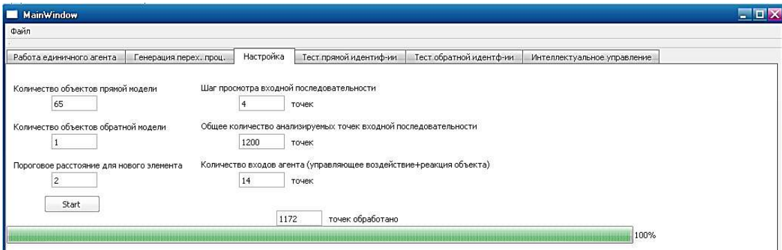
Рис. 7. Однократный просмотр точек переходного процесса с заданной дискретностью, настройка мультиагентной системы
