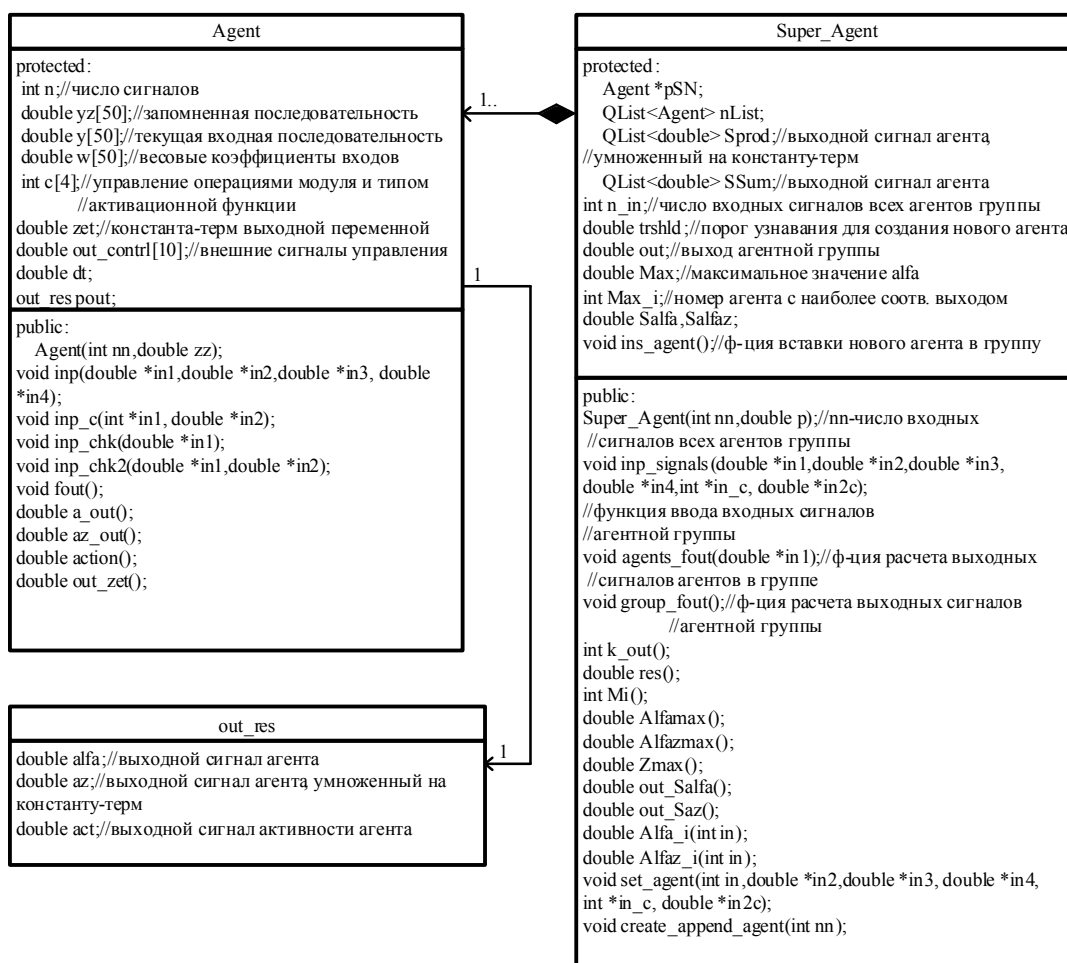
Рис. 3. UML-диаграмма классов тестовой мультиагентной системы
