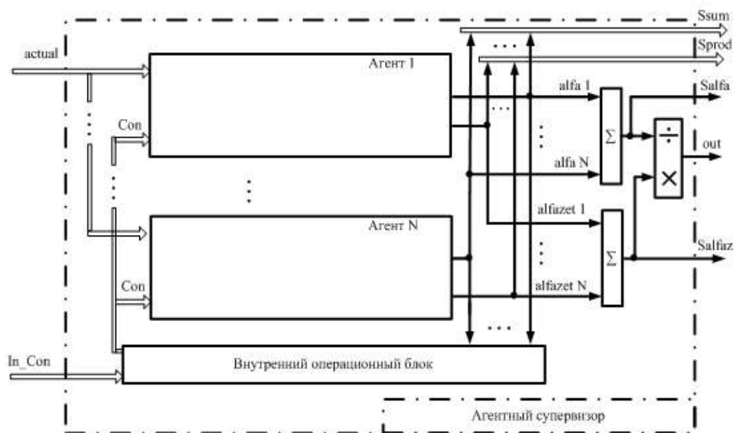
Рис. 2. Структура агентной группы с супервизором
