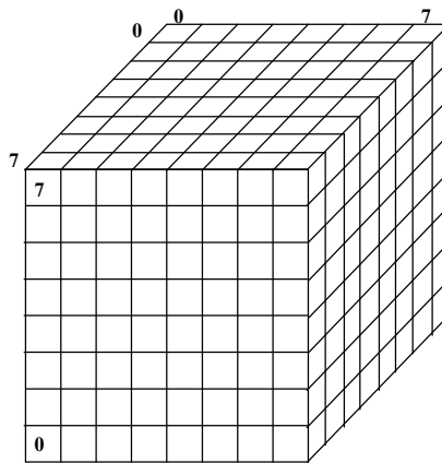
Рис. 2. Битовый куб
