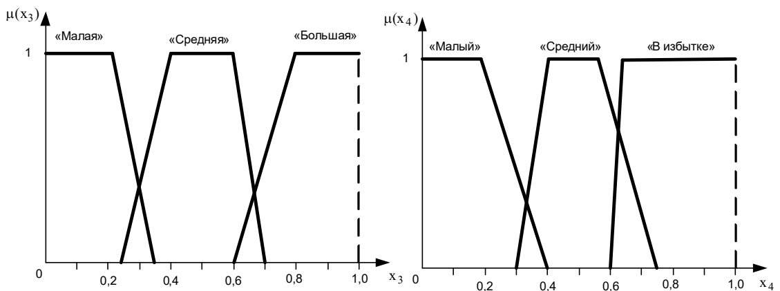
Рис. 3. Модель функции принадлежности для нечеткой переменной x_3 – оценка перспектив длительности простоя единицы основного оборудования
