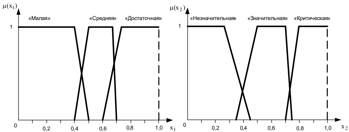
Рис. 1. Модель функции принадлежности для нечеткой переменной x_1 – степень выполнения плана
