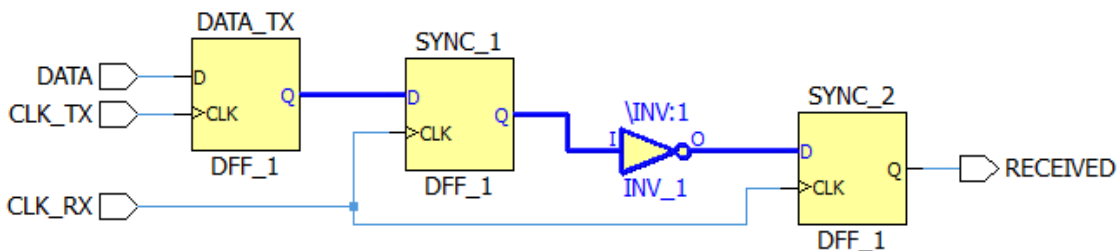
Рис. 7. Комбинационный элемент, нарушающий классический 2DFF-синхронизатор
