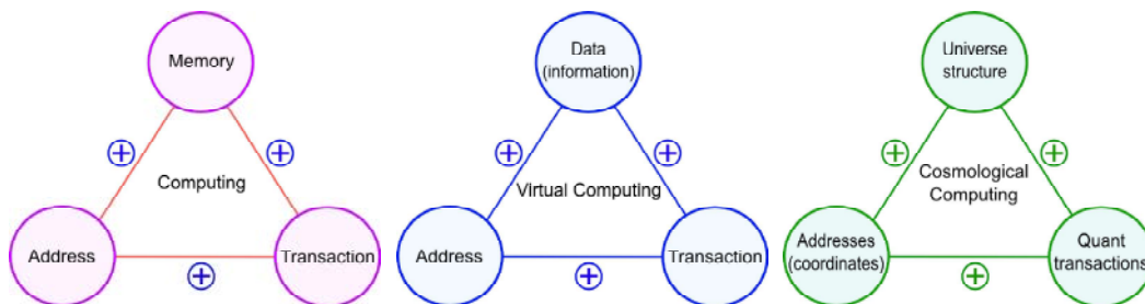
Рис. 3. Модель МАТ-компьютеринга
